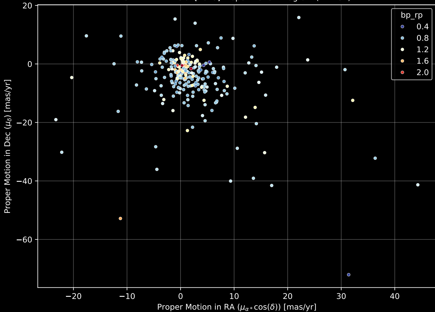
GALAH DR4 Field: [2845] Proper Motion Diagram (n= 254)
