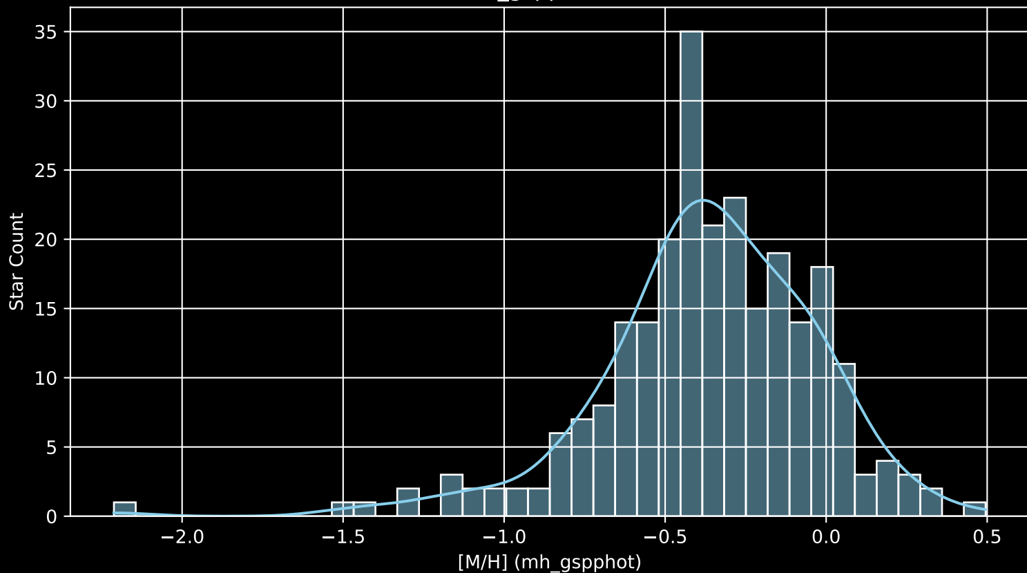
GALAH DR4 Field: [2845] [M/H] (mh_gspphot) (n= 254)
