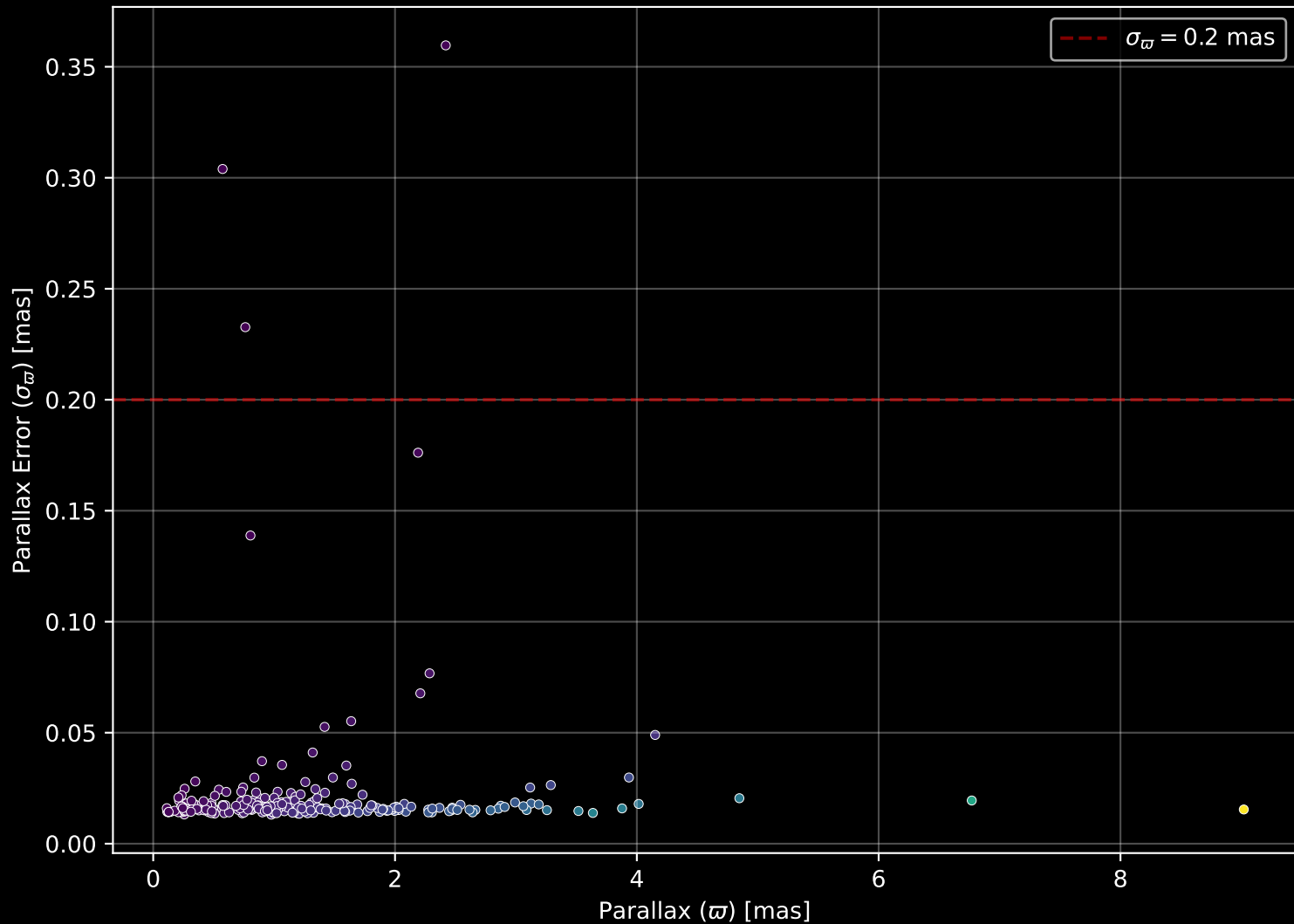
GALAH DR4 Field: [2845] Parallax Quality (n= 254)
