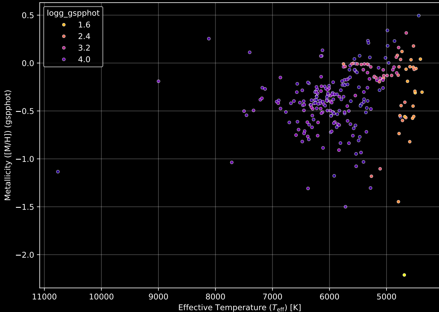
GALAH DR4 Field: [2845] Stellar Population Parameters (n= 254)
