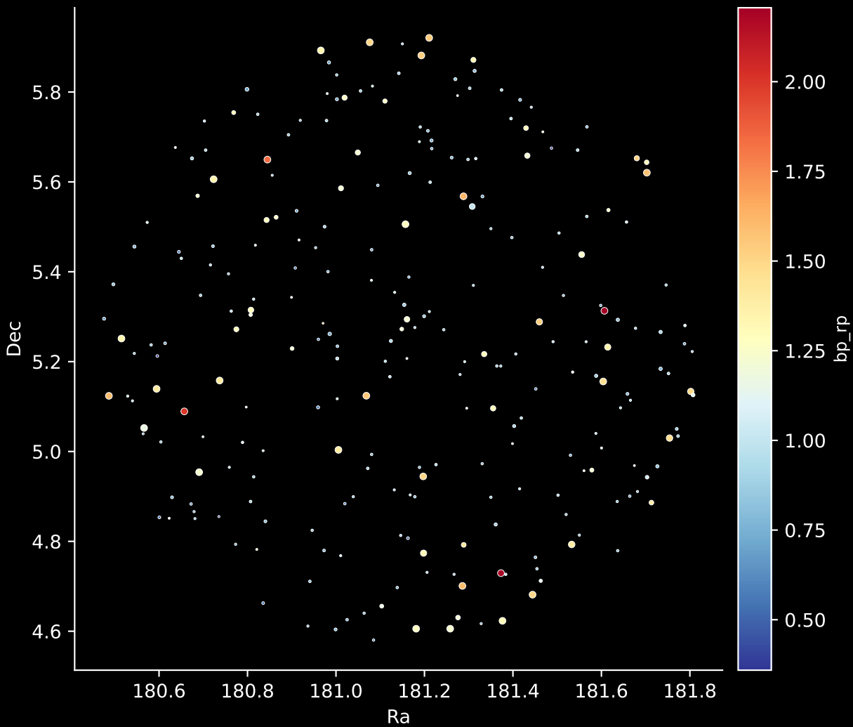
GALAH DR4 Field: [2845] Stars: 254
